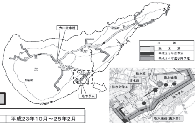
平成23年度の工事位置図
