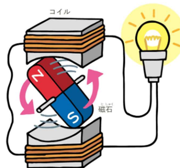
発電機の仕組み
